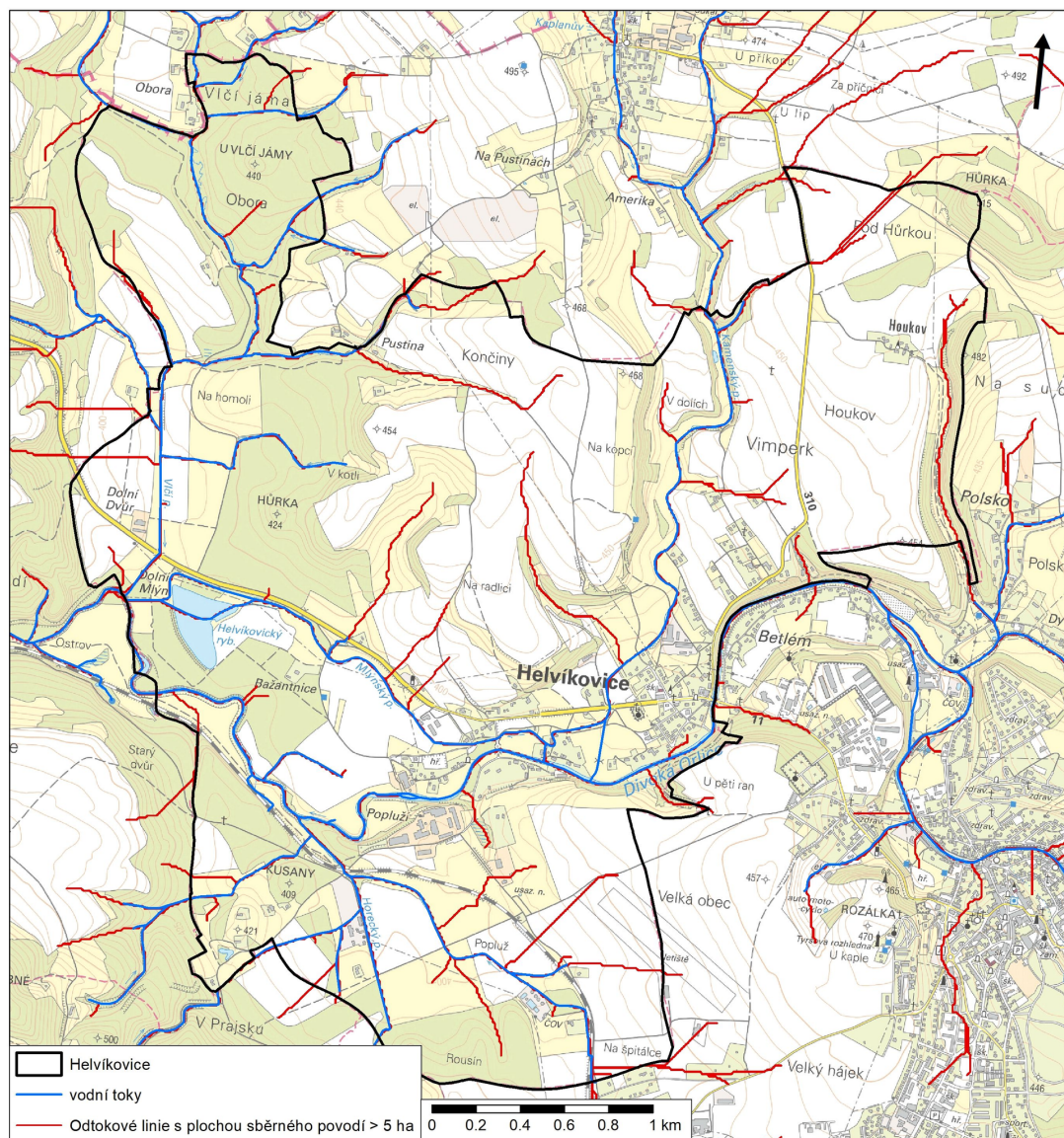
Obrázek 4: Odtokové linie s plochou sběrného povodí > 5 ha na území obce Helvíkovice
