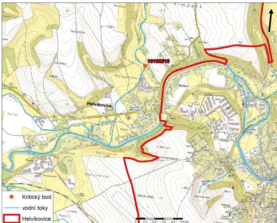
Obrázek 3: Zhodnocení vzniku přívalových povodní na území obce Helvíkovice metodou kritických bodů
